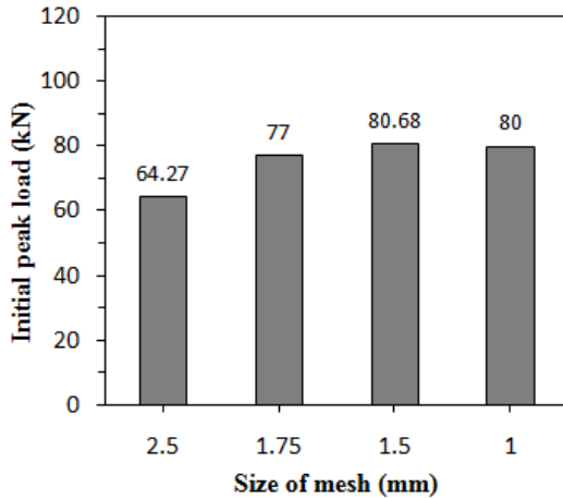
شکل ۸- همگرایی نیروی پیک اولیه برحسب اندازه مش برای لوله استوانه‌ای پر شده از فوم با آغازگر ۲۰mm
