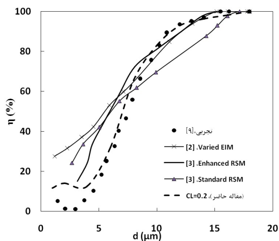
شکل ۱۳- مقایسه راندمان قطره‌گیری به‌دست آمده از شبیه‌سازی فعلی با نتایج به‌دست آمده قبلی برای سرعت ۲ (m/s) و عدد رینولدز ۲۱۹۲
