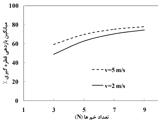
شکل ۱۹- میانگین بازدهی قطره‌گیری برحسب تعداد خم‌های مختلف برای سرعت‌های ۲(m/s) و ۵(m/s)
