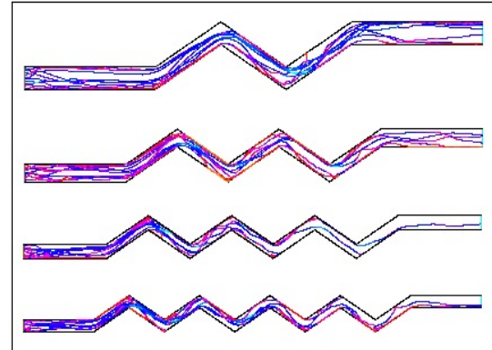
شکل ۱۶- نمایش اثر تعداد خم‌ها بر مسیر قطرات با سایز 8μm در جریان آشفته گاز با سرعت متوسط 2m/s
