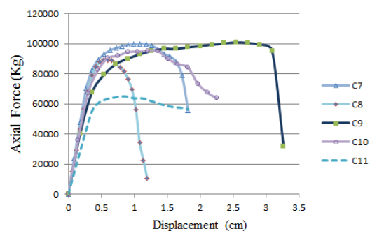
شکل ۸- منحنی‌های نیرو-جابجایی ستون‌های مرکب دو لایه
