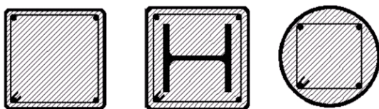
شکل ۱- ستون‌های SRC
