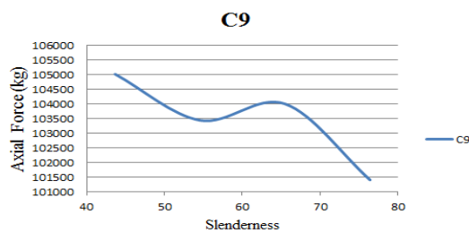
شکل ۱۲- اثر لاغری بر ظرفیت باربری ستون C9
