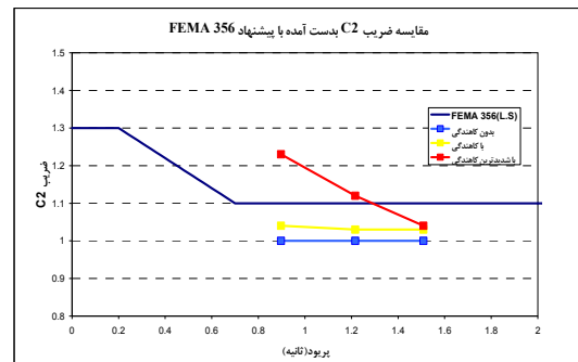
شکل ۳- مقایسه ضرایب C2 به دست آمده با FEMA356 [۱۴]
