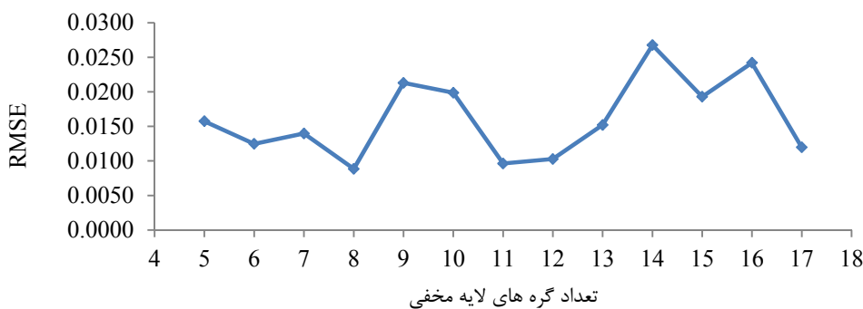
شکل ۱۲- جذر خطای میانگین مربعات به‌ازای تعداد گره‌های لایه مخفی در سیستم لایه‌بندی رسی
