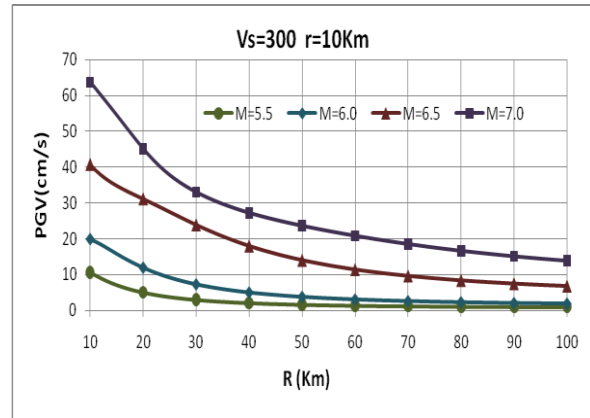
شکل ۱۰- نتایج سرعت ماکزیمم برای بزرگای مختلف (Reverse-Oblique Mechanism)
