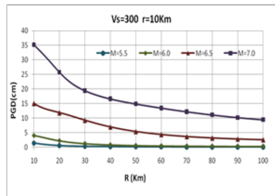
شکل ۱۱- نتایج تغییر مکان ماکزیمم برای بزرگای مختلف (Reverse-Oblique Mechanism)
