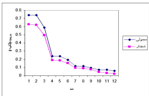
شکل ۱۲- نمودار پریود در ۱۲ مد اول
