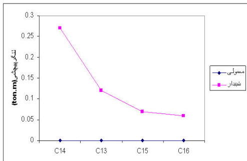
شکل ۱۱- نمودار لنگر پیچشی ستون‌های طبقه اول
