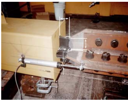
شکل ۳، نمایش قسمت محصور نشده هسته فولادی [۴]
